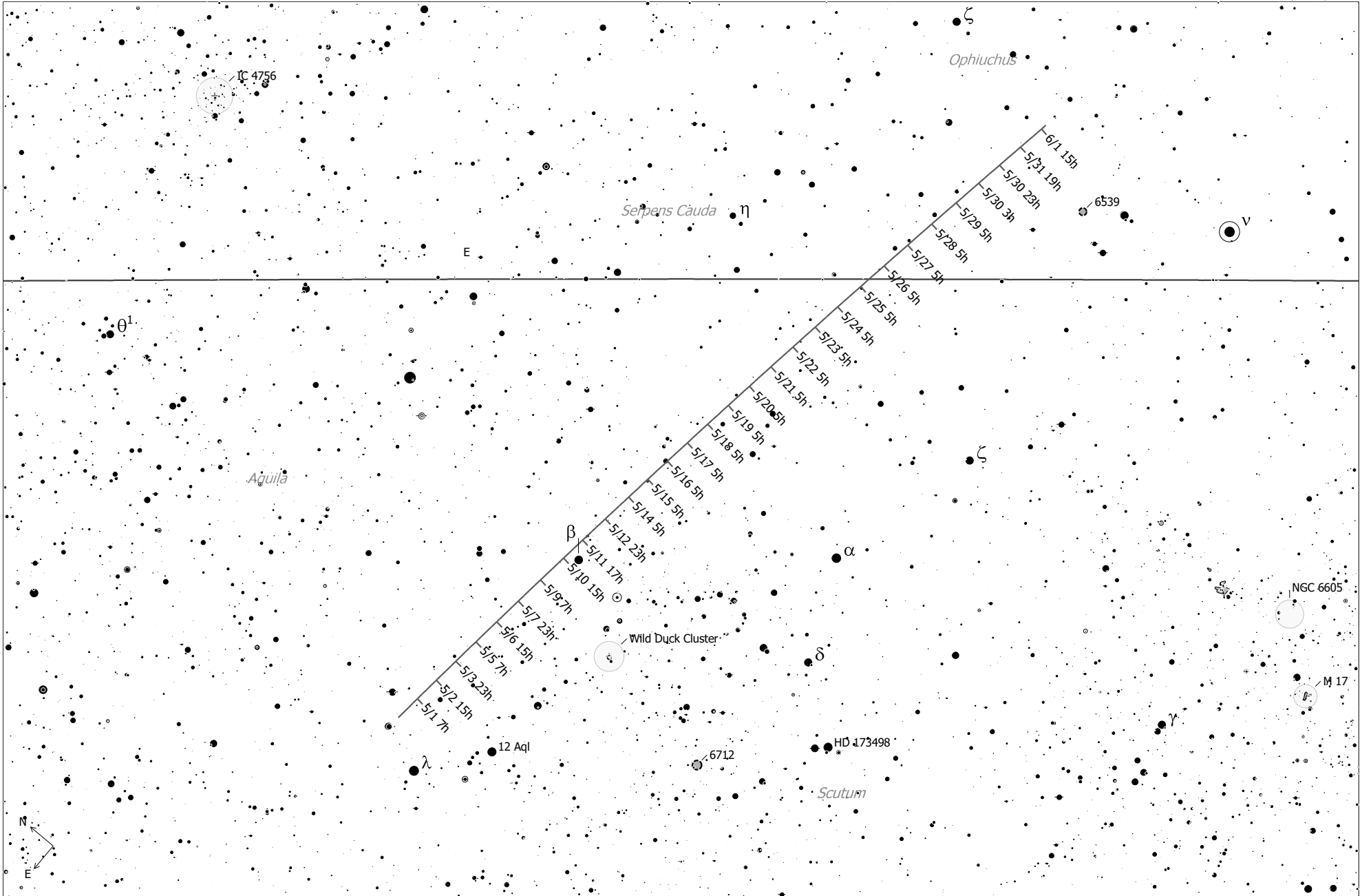
C/2023 R1 (PANSTARRS) (Comet)
